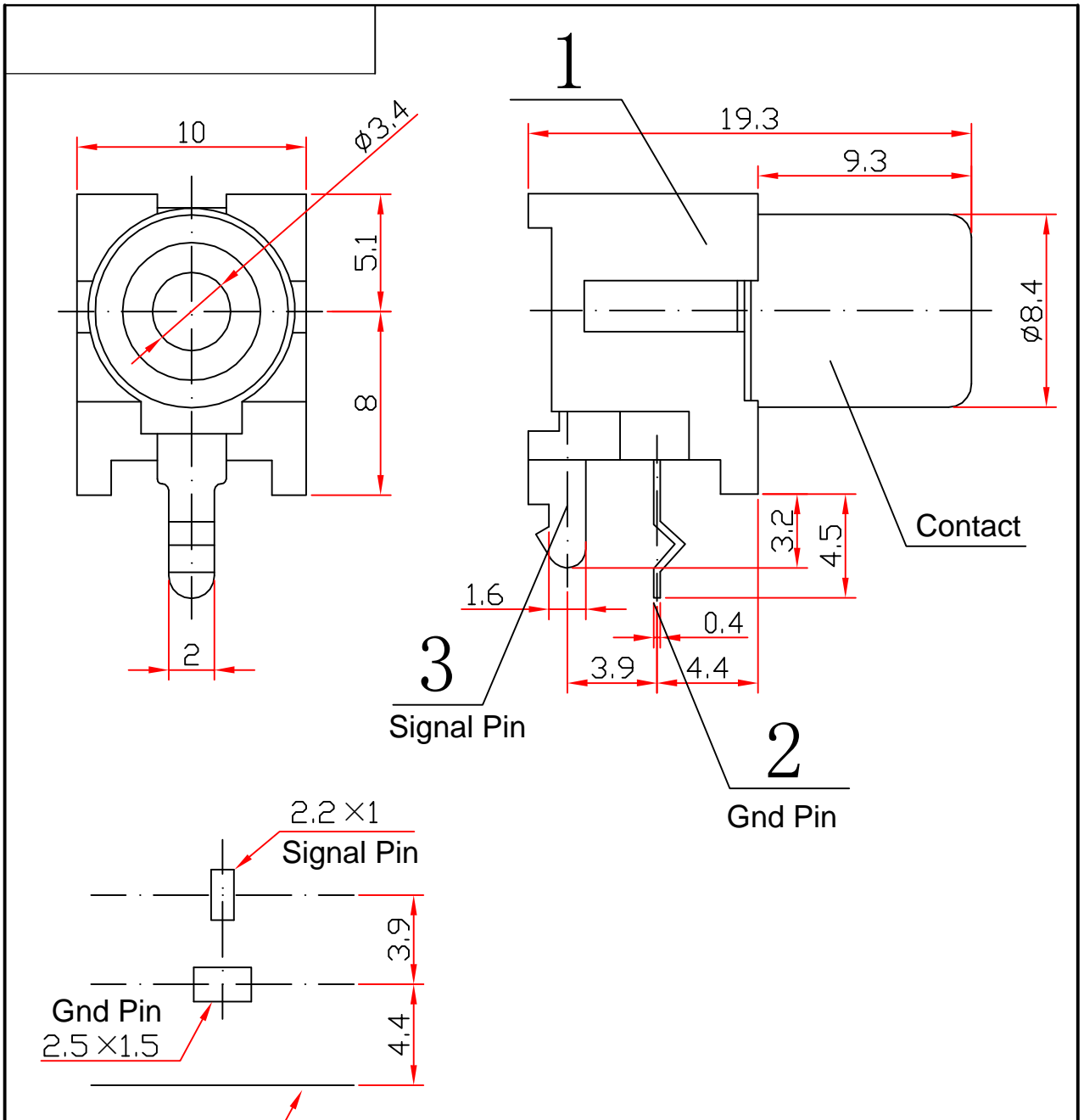
PCB Edge 印制电路板开孔尺寸
