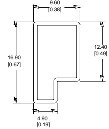
注: 单位 (Unit) : mm[inch] 未注明公差: x.x±0.5mm[x.x±0.020inch] 0.x±0.2mm[0.x±0.008inch] 管长: 220mm[8.66inch] 包装数量: 10pcs 内盒: 235*160*82mm 包装: 9管*5层 外箱: 335*225*280mm 包装: 6盒*1箱
