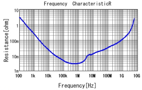
■ GRM188C80J106MEA6 R DCOV, 25degC
