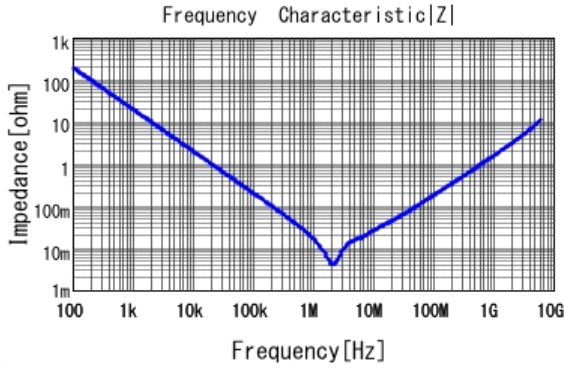
■ GRM188C80J106MEA6 |Z| DCOV, 25degC
