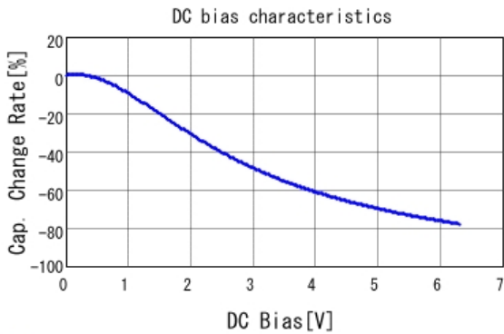
■ GRM188C80J106MEA6 C-DC bias capchange, 25.0degC, AC0.
