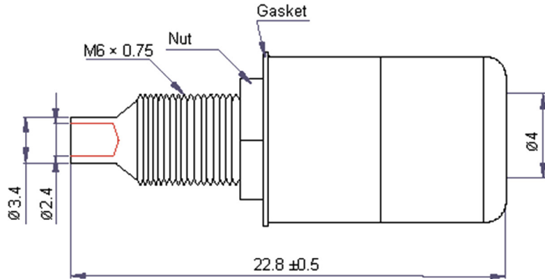
Dimensions : Millimetres
