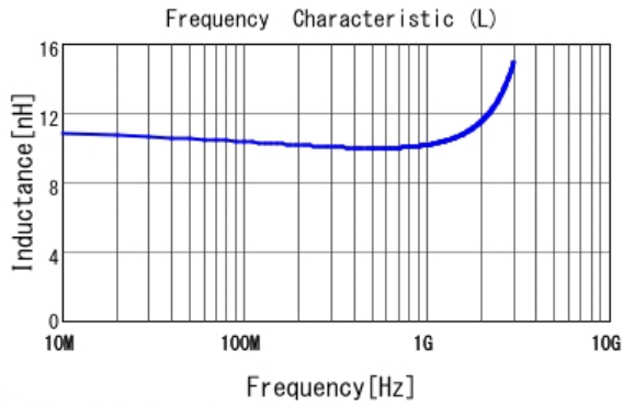
■ LQP03TN10NJZ2 L
