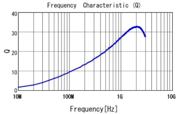
■ LQP03TN10NJZ2 Q
