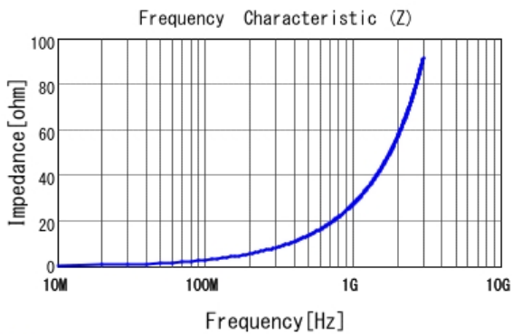
■ LQP03TQ4N3H02 |Z|
