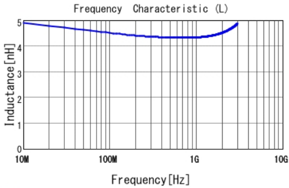
■ LQP03TQ4N3H02 L
