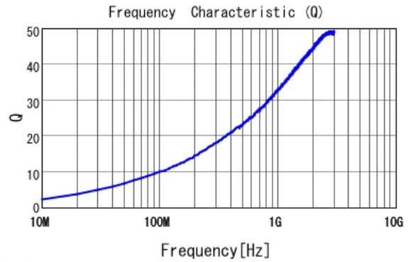
■ LQP03TQ4N3H02 Q
